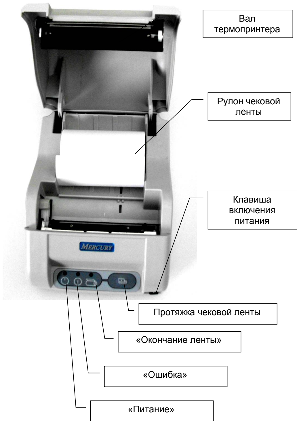
Рисунок 1. Внешний вид ККТ
